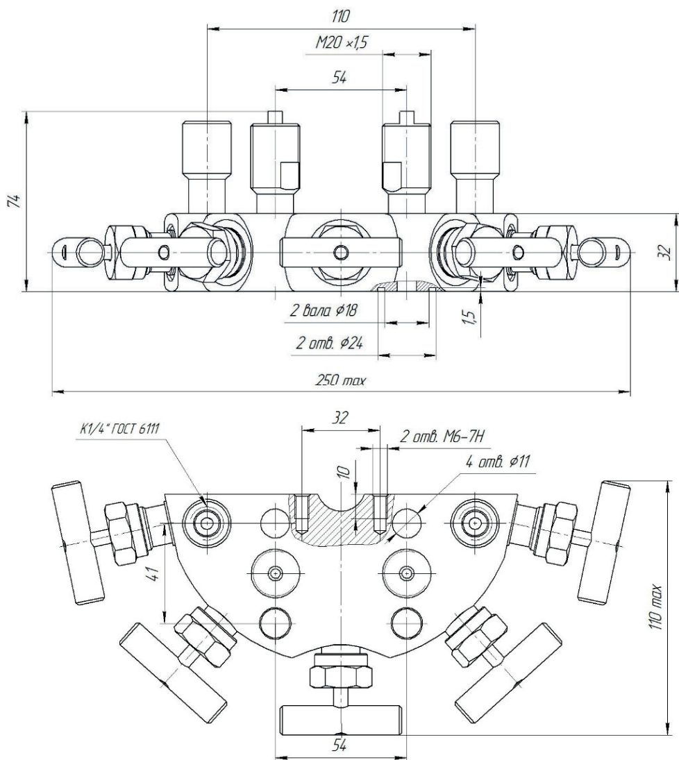
Рисунок А.26 — Блок клапанный БКН5-15
