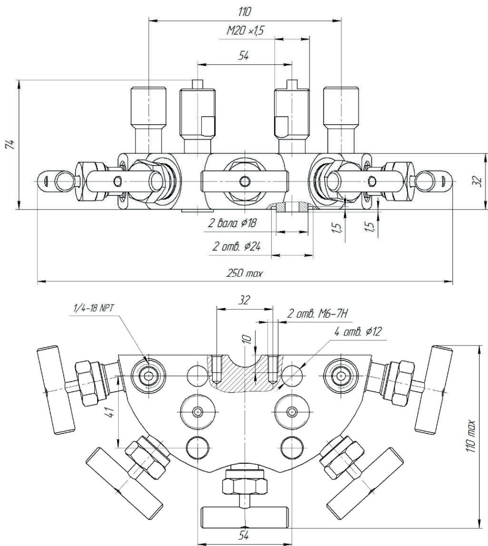
Рисунок А.24 — Блок клапанный БКН5-115-08
