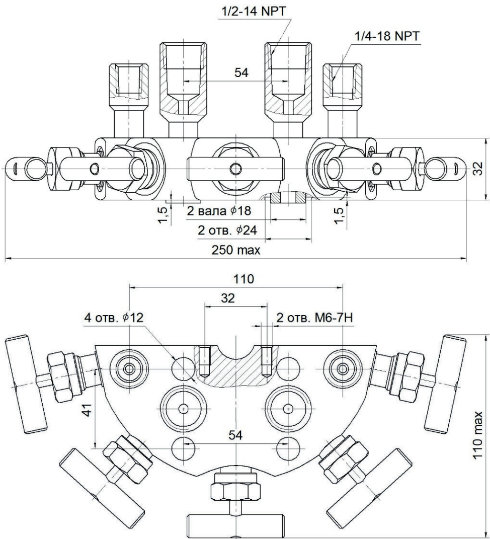
Рисунок А.23 — Блок клапанный БКН5-115-06
