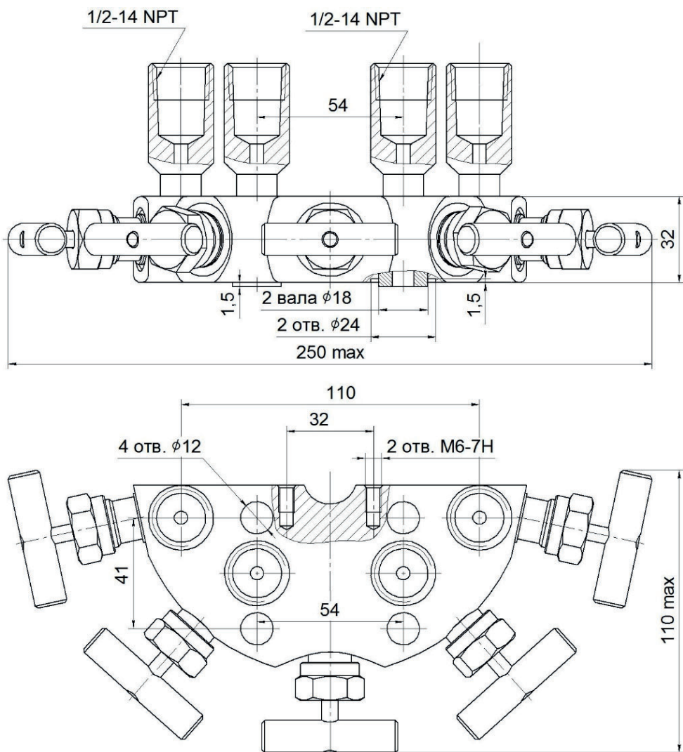
Рисунок А.22 — Блок клапанный БКН5-115-03
