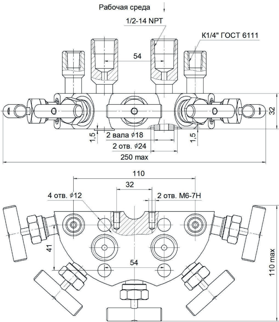
Рисунок А.21 — Блок клапанный БКН5-115-02
