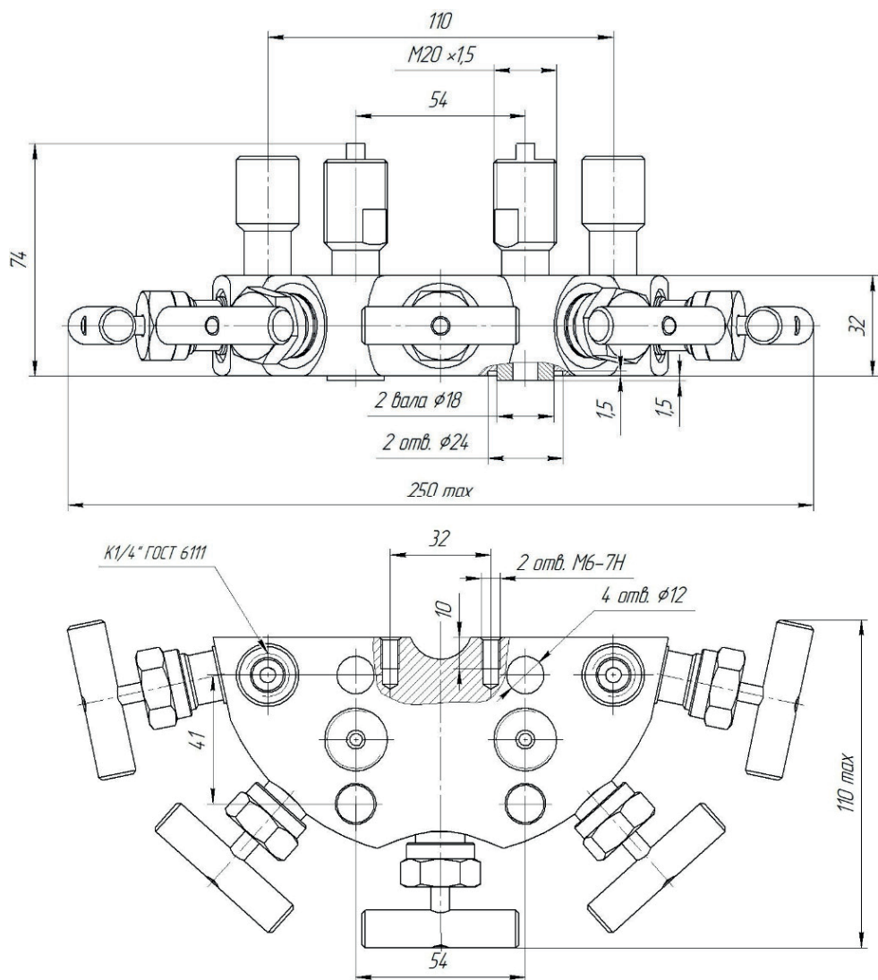
Рисунок А.19 — Блок клапанный БКН5-115
