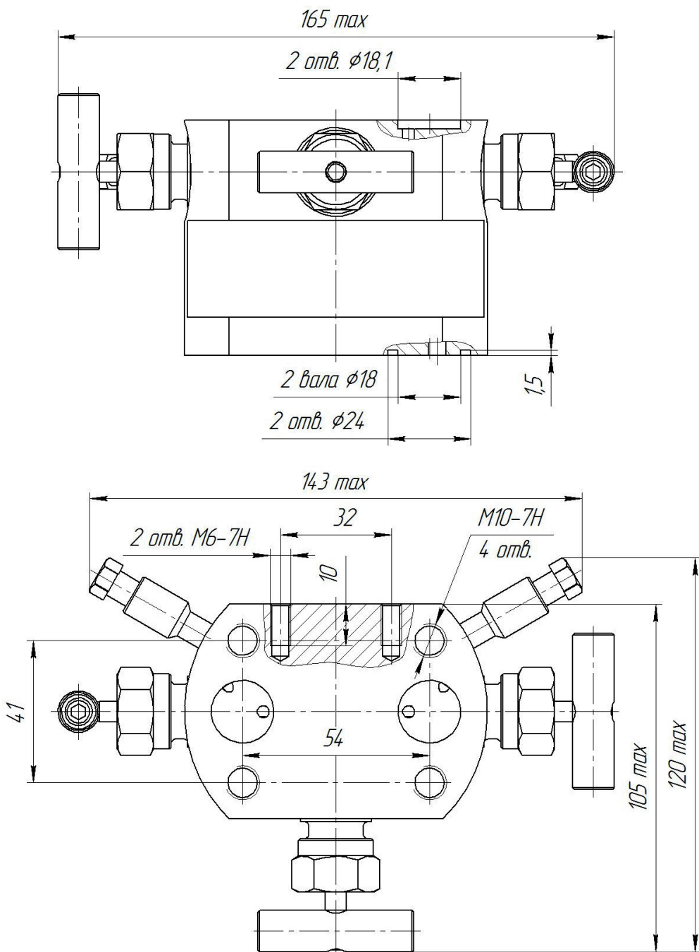
Рисунок А.2 — Блок клапанный БКНЗ-4-00
