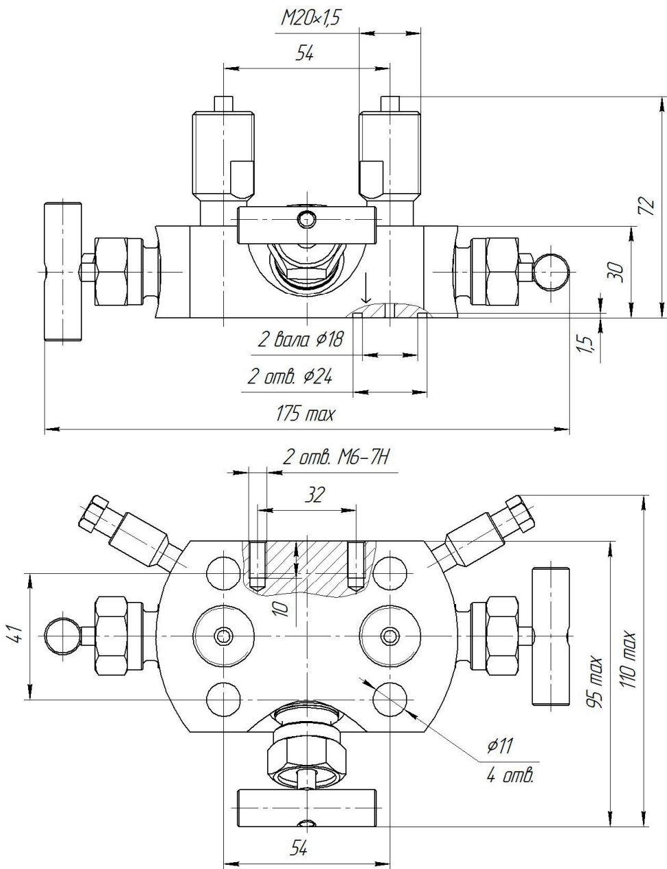
Рисунок А.8 — Блок клапанный БКНЗ-11-21
