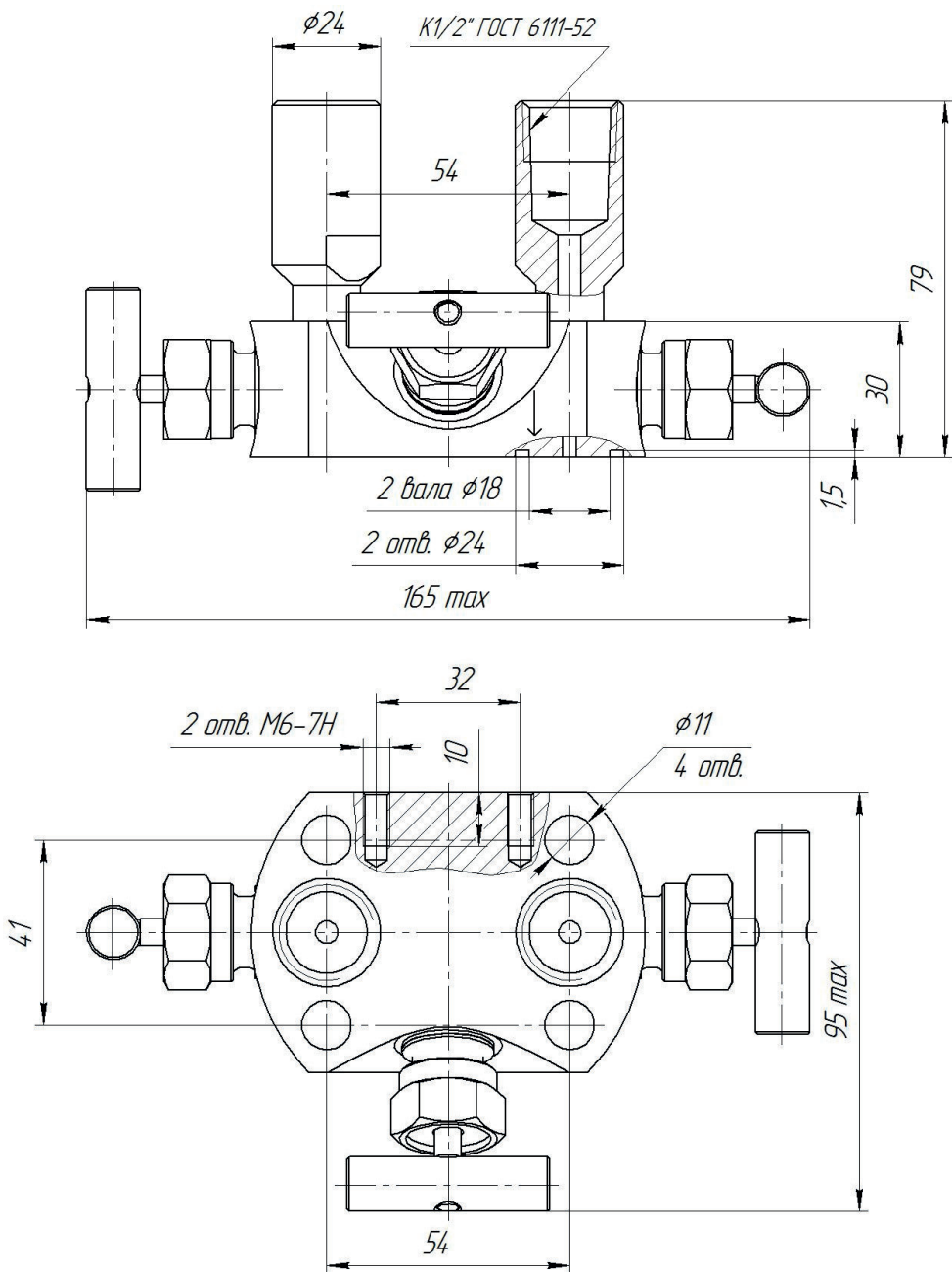
Рисунок А.6 — Блок клапанный БКНЗ-11-10
